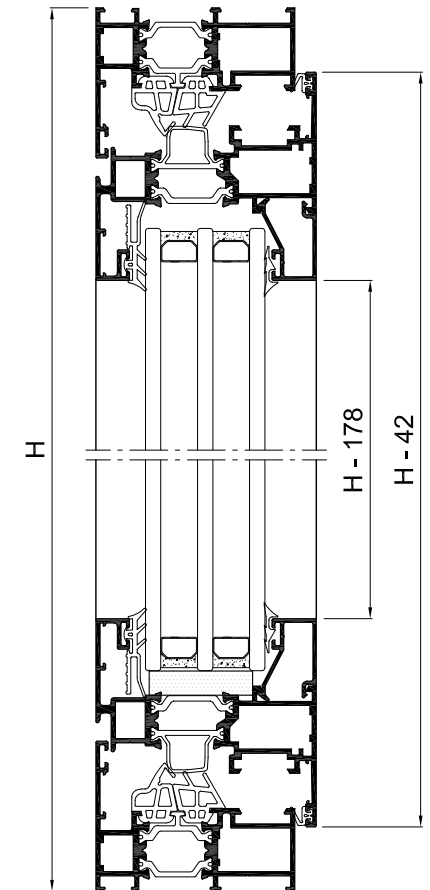
Sección B-B'
